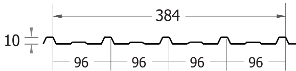
TYPE 5S
