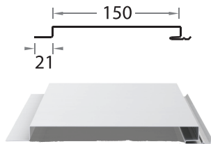
Spandrel A
