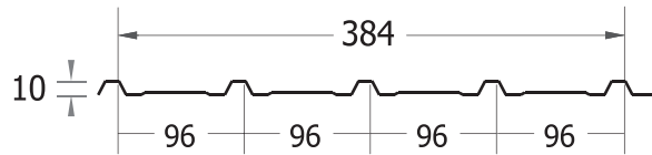
TYPE 5RIB
